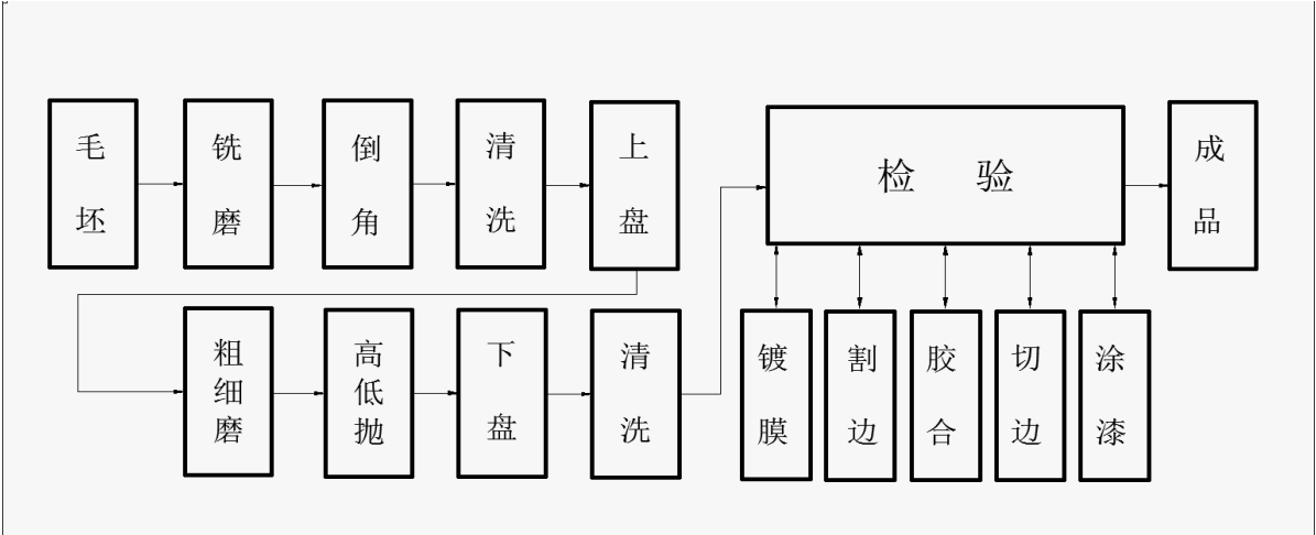
图 3-3 工艺布局图
